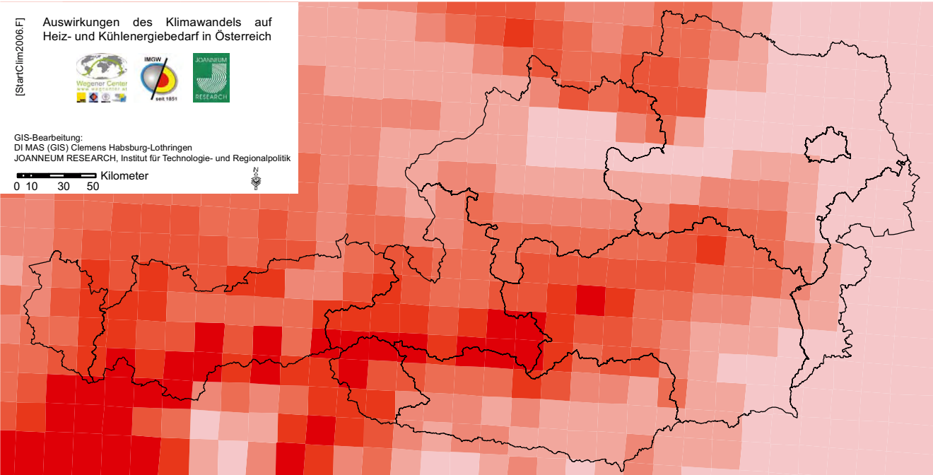
Abnahme der Heizgradtage 1981-1990 vs. 2041-2050 Heizgradtage (HGT)
