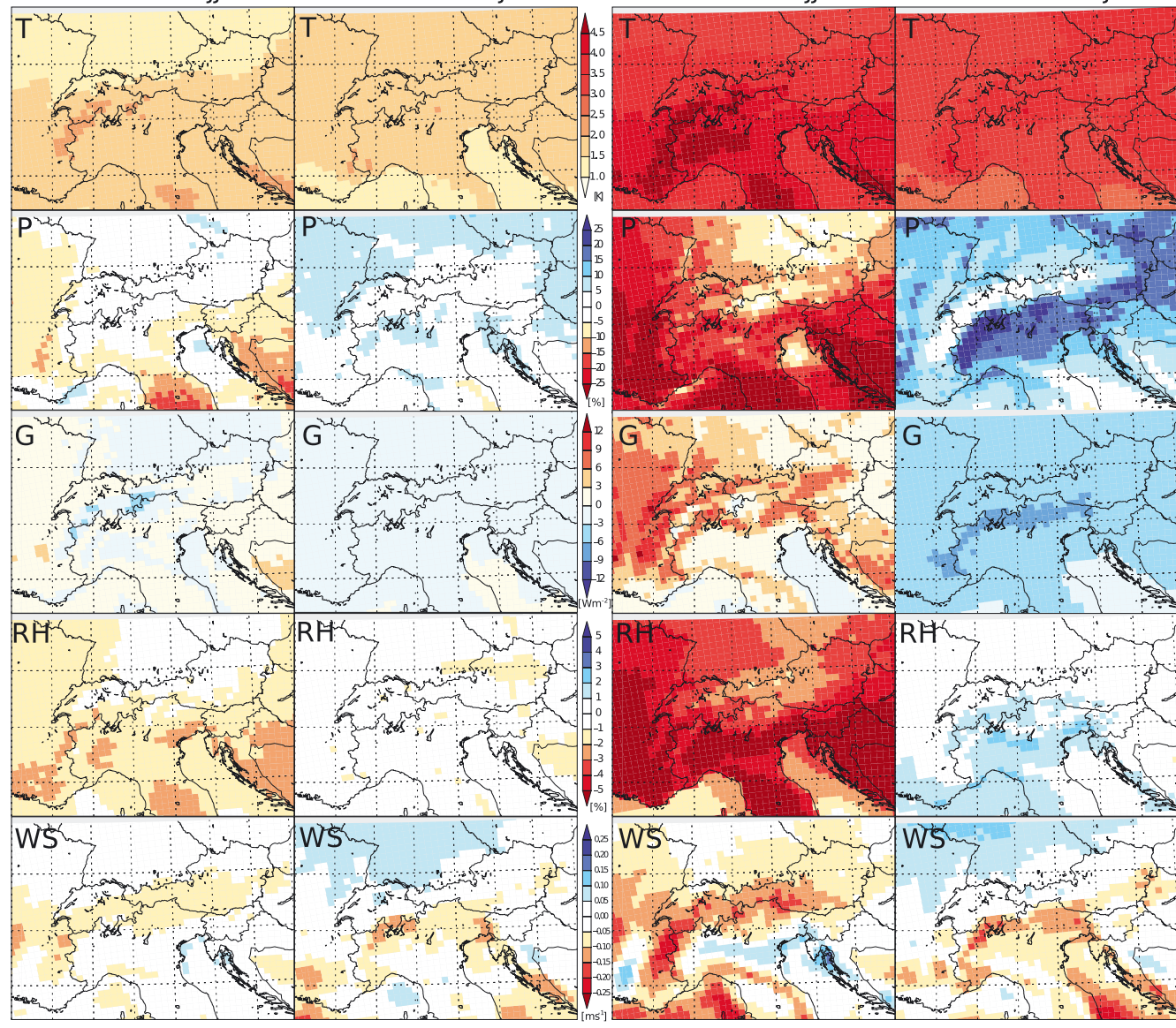
2012-2050 JJA
