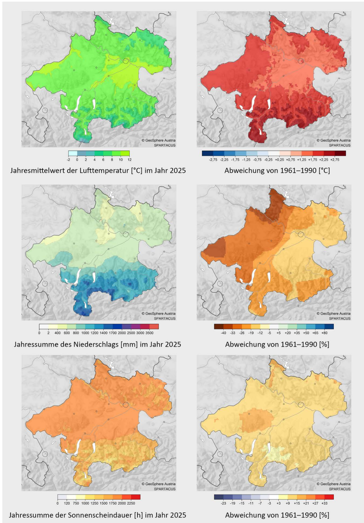
Abbildung 4: Räumliche Verteilung der Jahreswerte 2025 von Lufttemperatur (oben), Niederschlagssumme (Mitte) und Sonnenscheindauer (unten) in Oberösterreich als Absolutwerte (links) und als Abweichungen vom Mittelwert des Bezugszeitraumes 1961–1990 (rechts).
