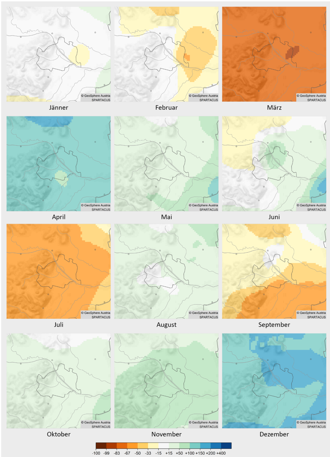
Abbildung 6: Räumliche Verteilung der Abweichungen der Monatssummen des Niederschlags in % im Jahr 2023 vom Mittelwert des Bezugszeitraumes 1961–1990 in Wien.
