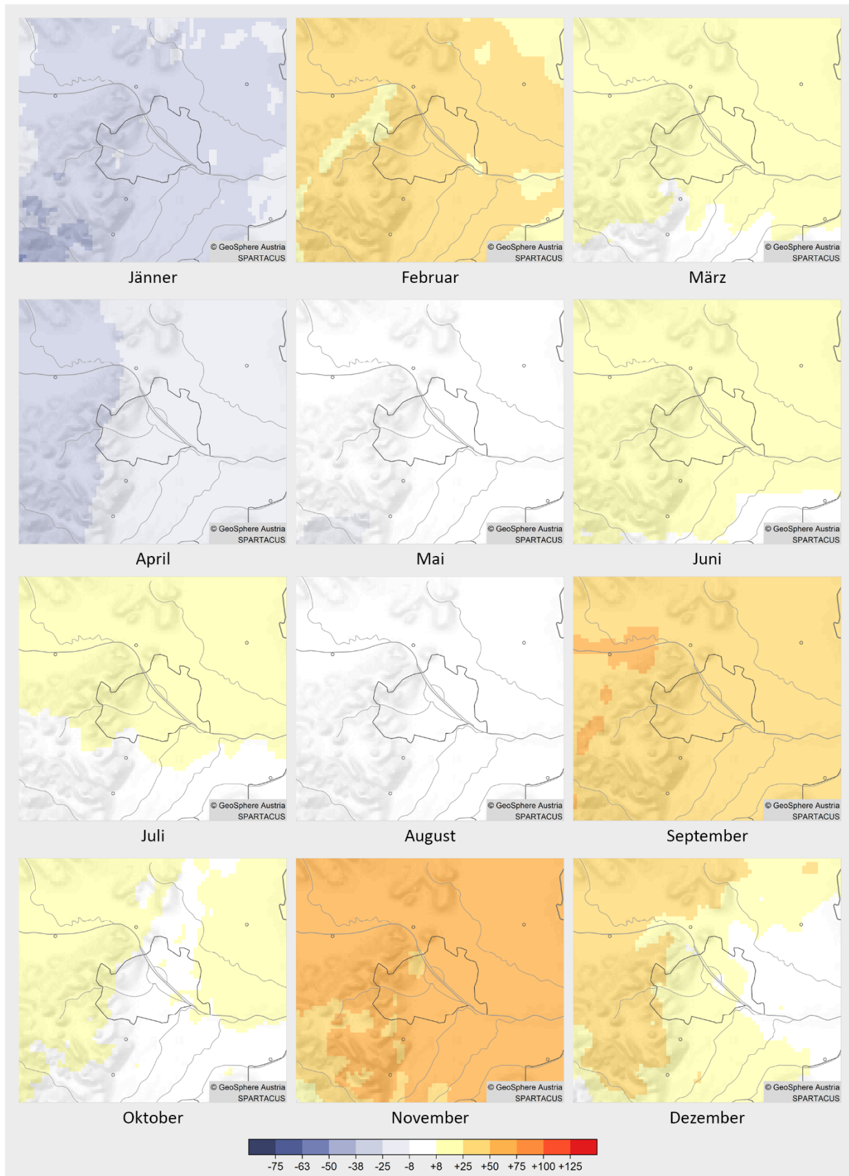
Abbildung 7: Räumliche Verteilung der Abweichungen der Monatssummen der Sonnenscheindauer in % im Jahr 2023 vom Mittelwert des Bezugszeitraumes 1961–1990 in Wien.
