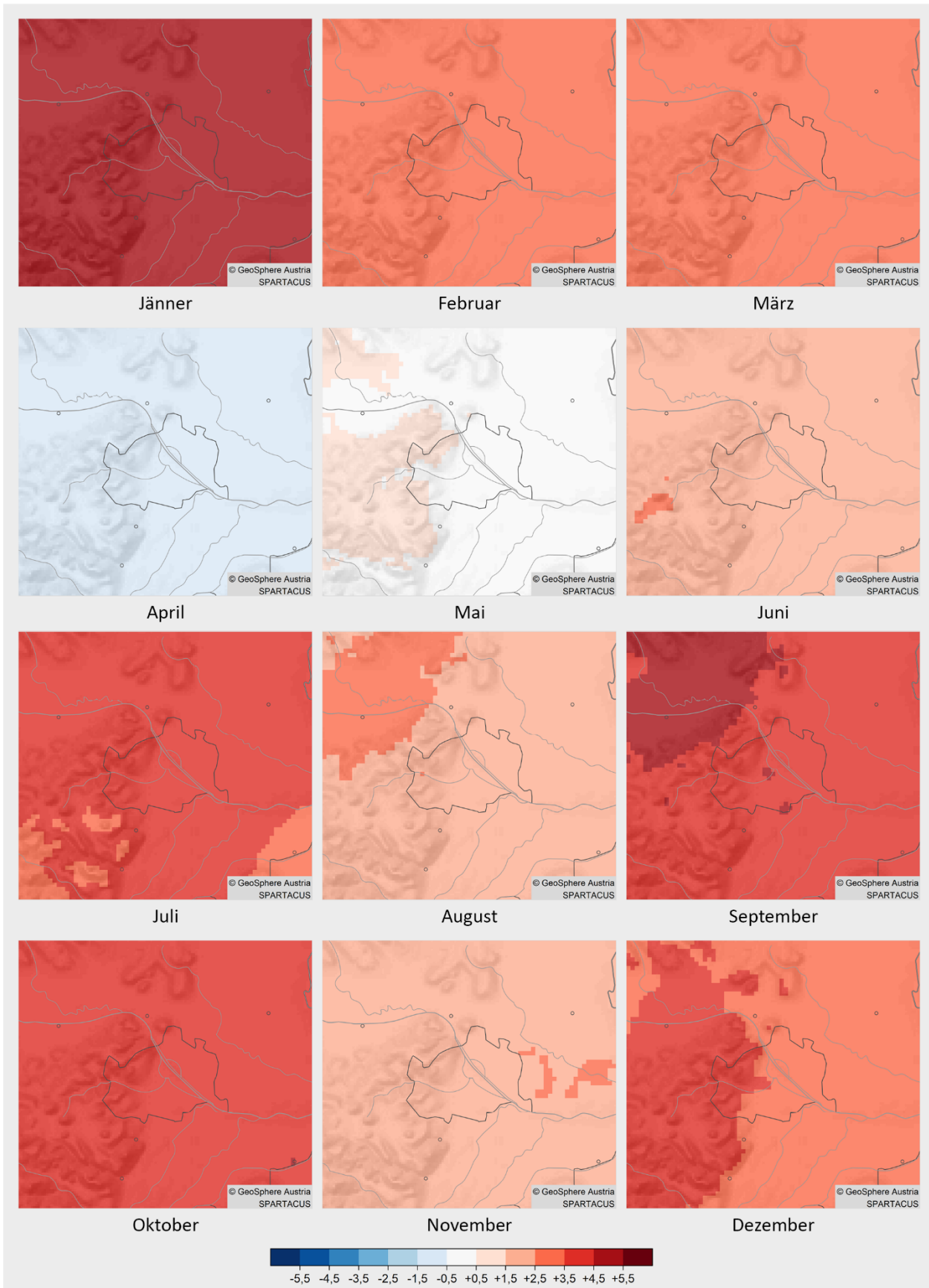
Abbildung 5: Räumliche Verteilung der Abweichungen der Monatsmittelwerte der Lufttemperatur in °C im Jahr 2023 vom Mittelwert des Bezugszeitraumes 1961–1990 in Wien.
