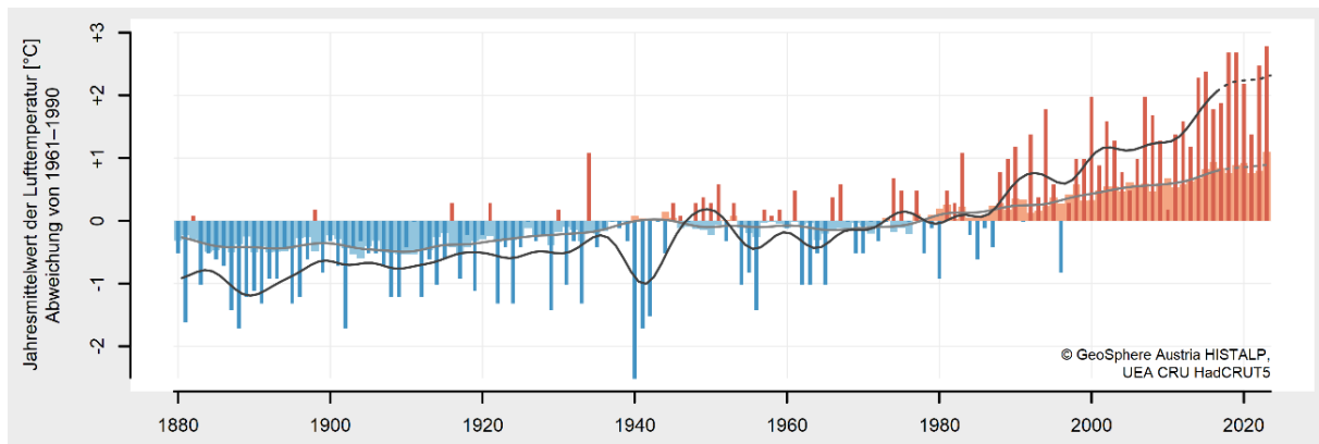
Abbildung 9: Langfristige Entwicklung der Jahreswerte der Lufttemperatur global und in Wien von 1880 bis 2023. Dargestellt sind Abweichungen von den jeweiligen Mittelwerten des Bezugszeitraumes 1961–1990.
