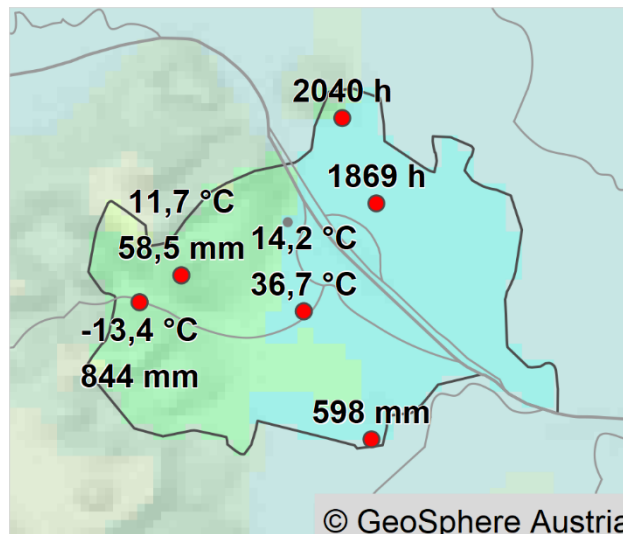
Abbildung 2: Räumlicher Überblick der an Klimastationen beobachteten Wetterextreme im Jahr 2023 in Wien.
