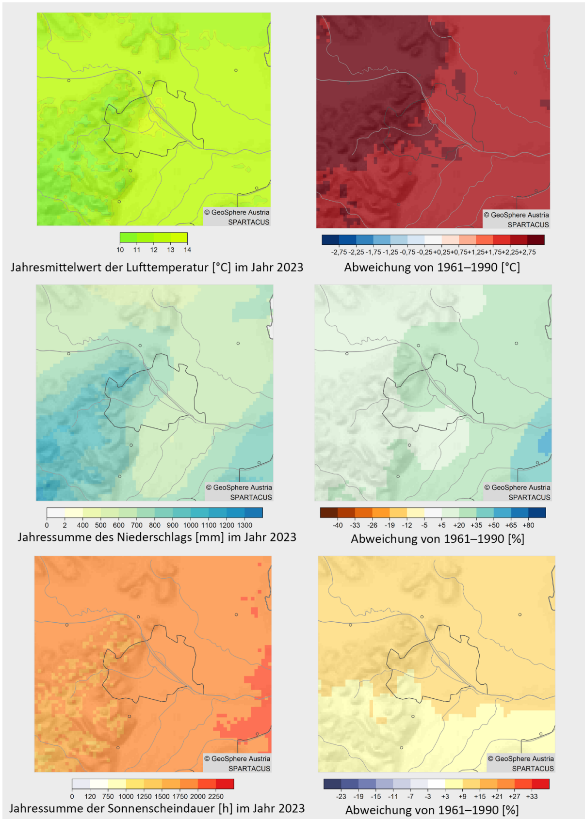
Abbildung 4: Räumliche Verteilung der Jahreswerte 2023 von Lufttemperatur (oben), Niederschlags- summe (Mitte) und Sonnenscheindauer (unten) in Wien als Absolutwerte (links) und als Abweichungen vom Mittelwert des Bezugszeitraumes 1961–1990 (rechts).
