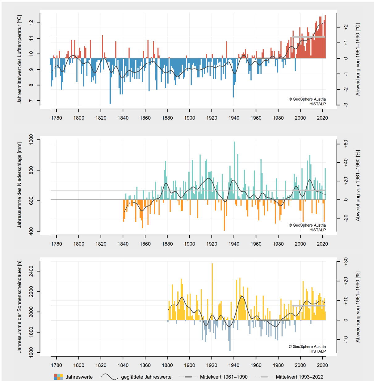
Abbildung 8: Langfristige Entwicklung der Jahreswerte von Lufttemperatur (oben), Niederschlags-summe (Mitte) Sonnenscheindauer (unten) in Wien vom Beginn instrumenteller Messungen bis 2023. Die Niveaus der Mittelwerte des Bezugszeitraumes 1961–1990 bzw. der letzten 30 Jahre 1993–2022 sind als dunkelgraue bzw. hellgraue Linien eingetragen.
