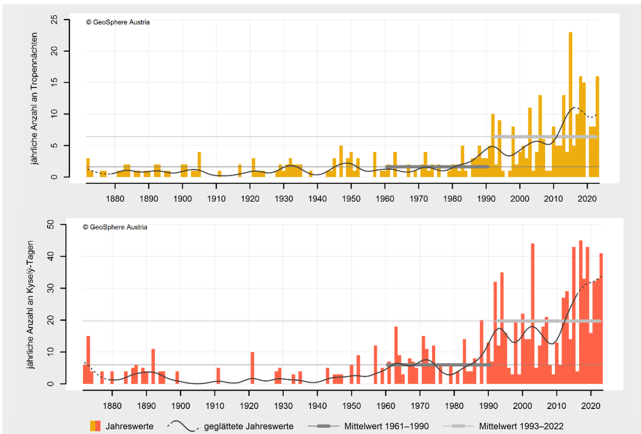
Abbildung 10: Entwicklung der jährlichen Anzahl an Tropennächten (oben) und Kysely-Tagen (unten) in Wien von 1948 bis 2023. Die Niveaus der Mittelwerte des Bezugszeitraumes 1961–1990 bzw. der letzten 30 Jahre 1993–2022 sind als dunkelgraue bzw. hellgraue Linien eingetragen.
