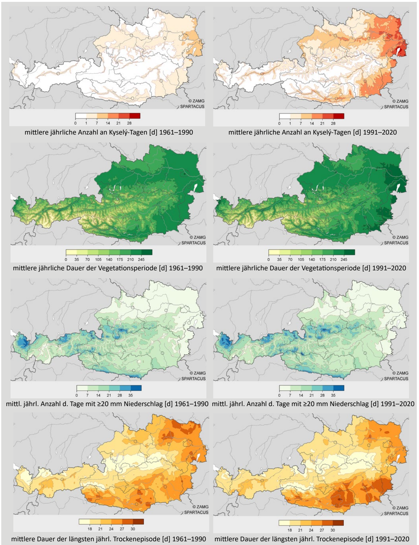
Abbildung 8: Räumliche Verteilung der mittleren Jahreswerte der Klimaindizes Hitzeperiode nach Kyselý (oben), Vegetationsperiode (Mitte oben), Starkniederschlagstage (Mitte unten) und Trockenepisode (unten) in den Bezugszeiträumen 1961–1990 (links) und 1991–2020 (rechts) in Österreich.
